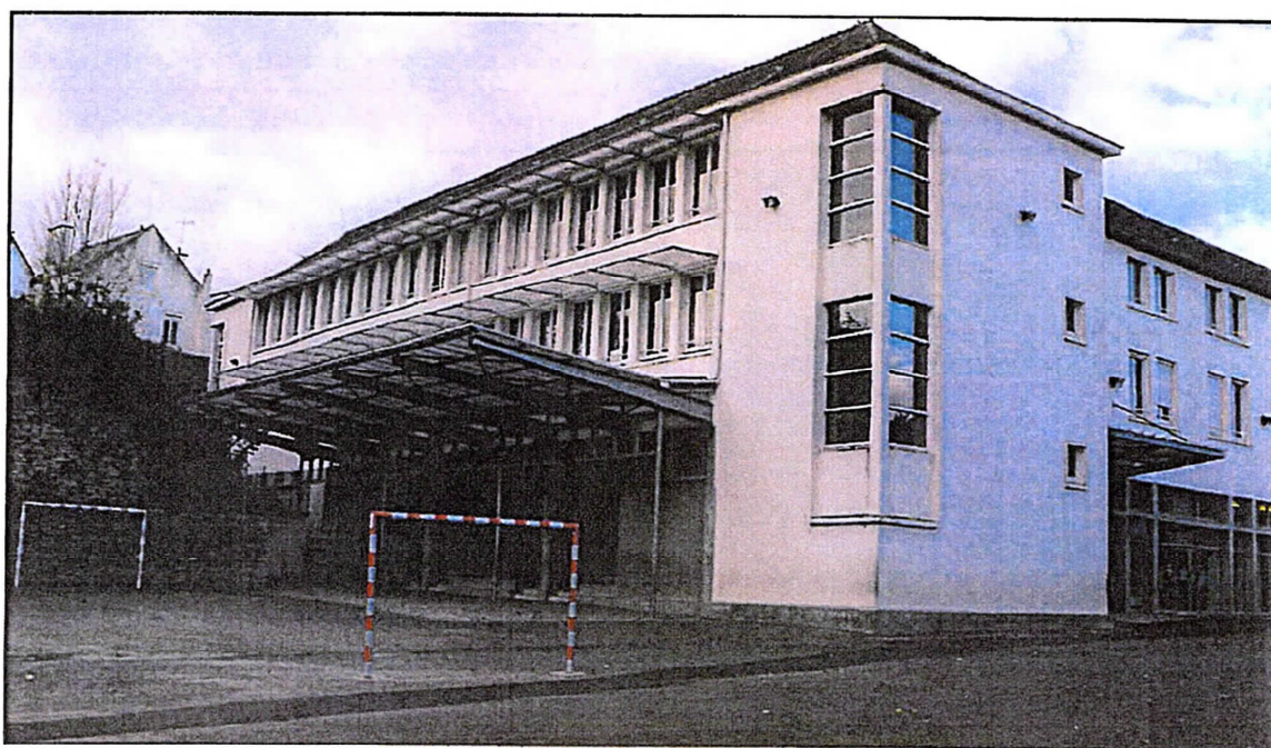
AUVENT DU PRÉAU OUVERT SUR LES VENTS DOMINANTS - HAUTEUR 6,00M
